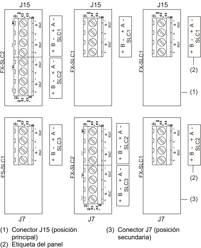
Figura 4: Configuraciones de número de SLC para paneles FX-1000
