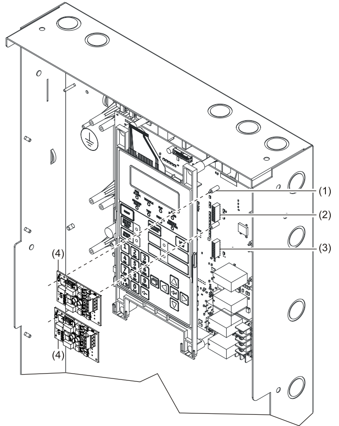
Figura 3: Instalación de una tarjeta FX-SLC1 en un panel FX-1000
