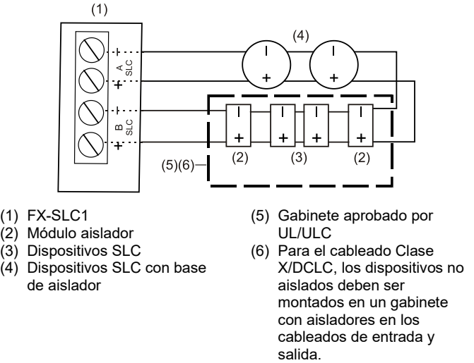
Figura 7: Cableado Clase X/DCLC [2]
