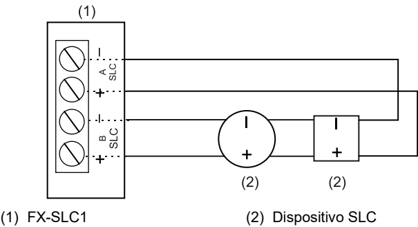
Figura 6: Cableado Clase A/DCLA [1]
