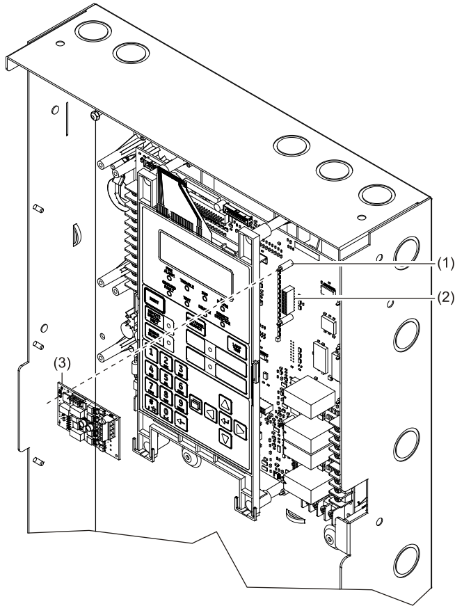
Figura 2: Instalación de una tarjeta FX-SLC1 en un panel FX-64
