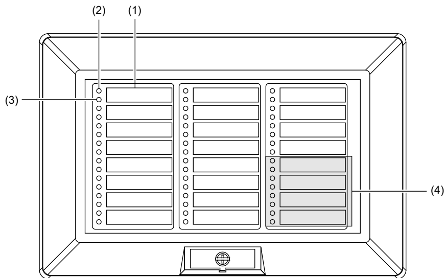
Figura 13: Controles e indicadores para RLED24-2 y RLED24R-2
