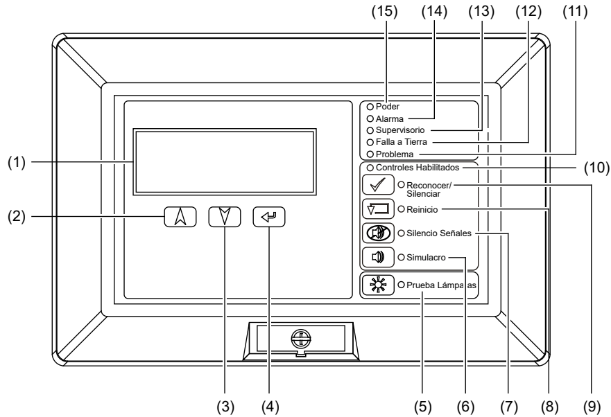
Figura 11: Controles e indicadores para anunciadores remotos LCD sin controles comunes
