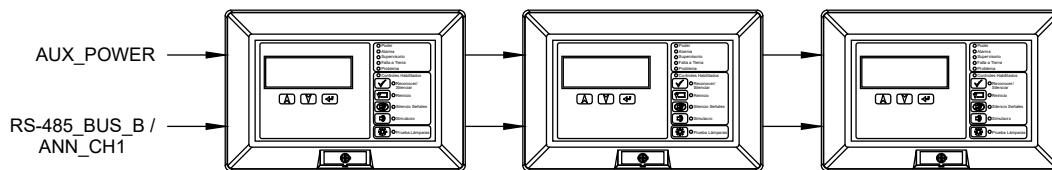
Figura 6: Cableado Clase B/DCLA redundante Típico
