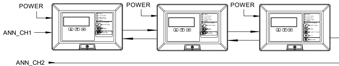
Figura 7: Cableado Clase A/DCLA Típico
